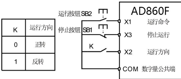
图 6-6 三线式模 2
