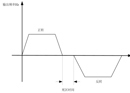
图 6-18 正反转死区时间示意图
