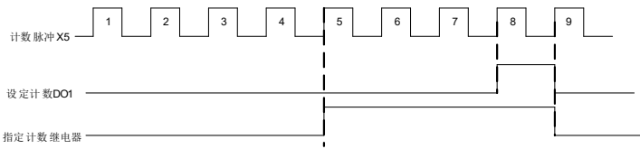
图 6-29 设定计数值给定和指定计数值给定示意图
