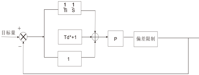
图 6-25 过程 PID 原理框图
