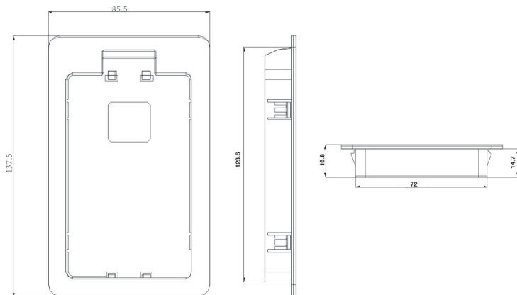
面板托架开孔尺寸：123.6mm * 72mm
