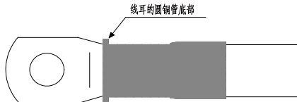
线缆导线露出导体套热缩管示意图
