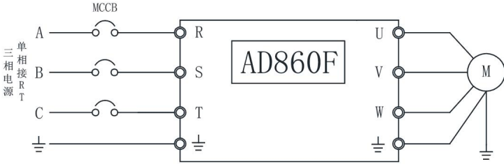
上图: 接简单运行线
